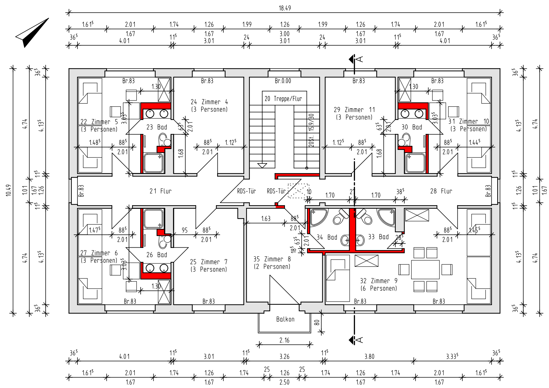
Grundriss Obergeschoss - Planung
